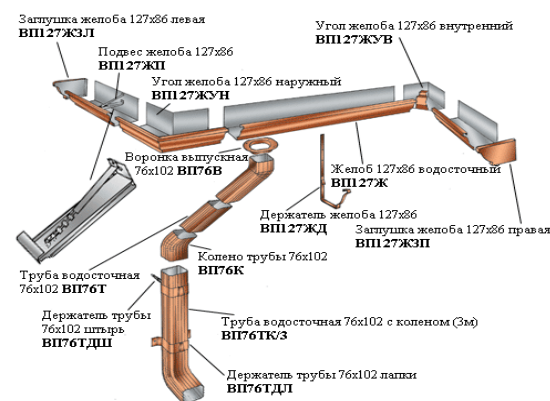
Водосточная труба
