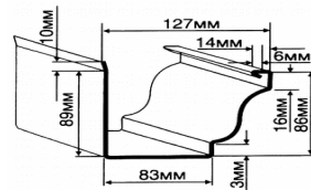
Желоб
